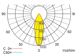
Leuchtmittel: 3W LED-Leiste
